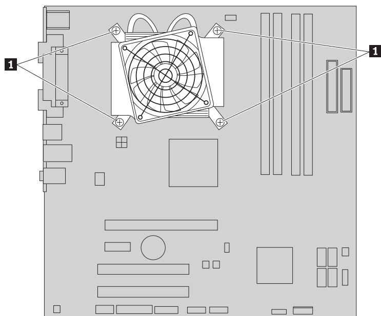
Figura 30. Scoaterea radiatorului fixat cu șuruburi
