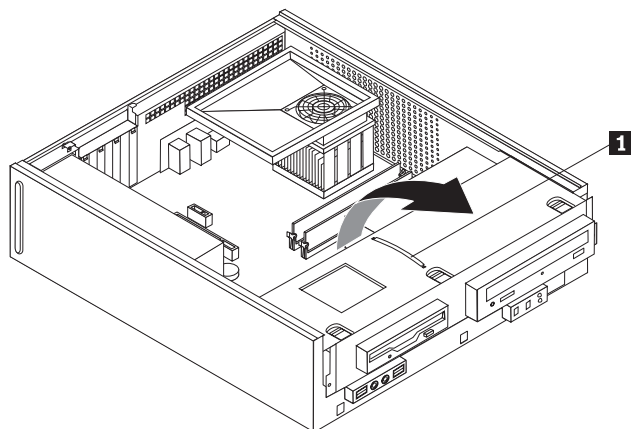
Figura 8. Înlăturarea ansamblului locașului de unitate
