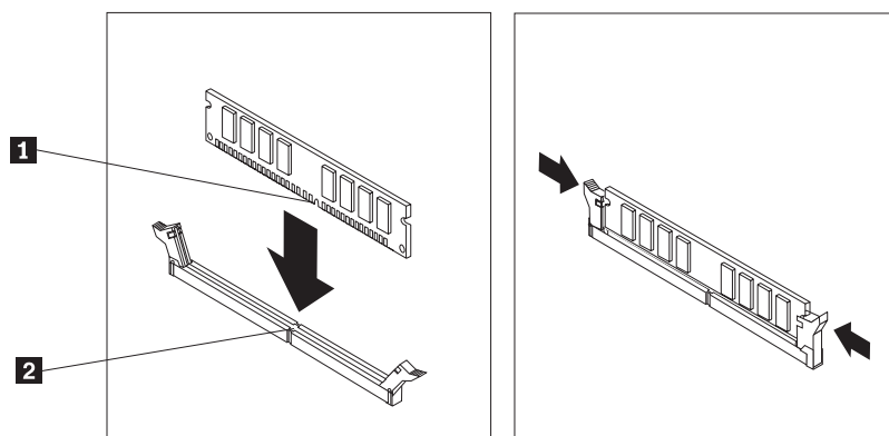
Figura 10. Poziționarea modului de memorie
