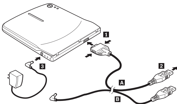
圖 1-1. 配置 1：自動電源（AC 整流器）配置
