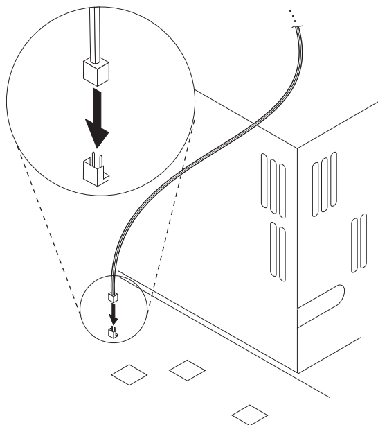
図 2-11. PC Wake on LAN 信号コネクター (2ピン)
