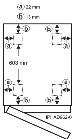
Figure 14. Emplacements des roulettes des modèles 05/54 et 14S/11
