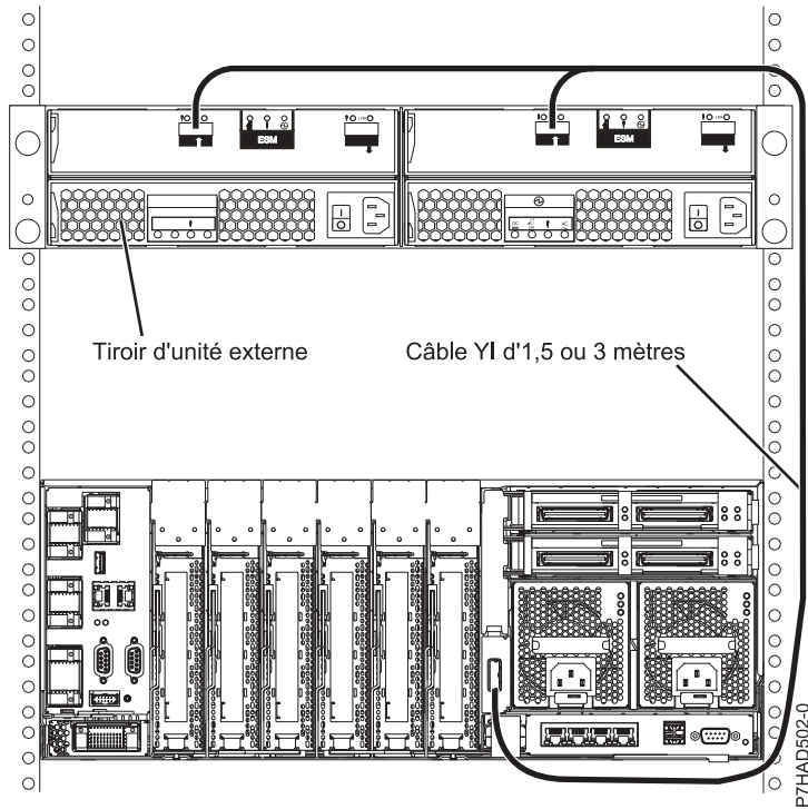
Figure 125. Connexion d'un port de carte SAS externe du système à un tiroir d'extension de disque (modèles 9117-MMB et 9179-MHB)
