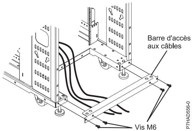
Figure 22. Barre d'accès aux câbles
