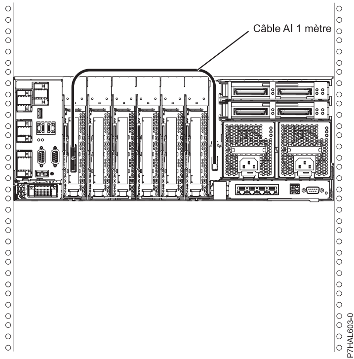
Figure 126. Connexion d'une carte SAS aux emplacements de disque SAS internes via un port SAS externe système
