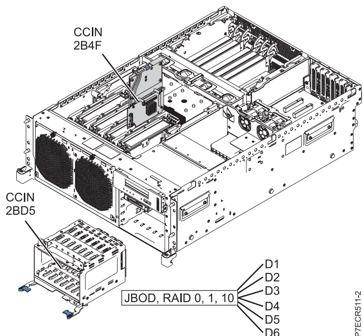
Figure 5. Adaptateur SAS intégré dans un fond de panier d'unité à deux voies
