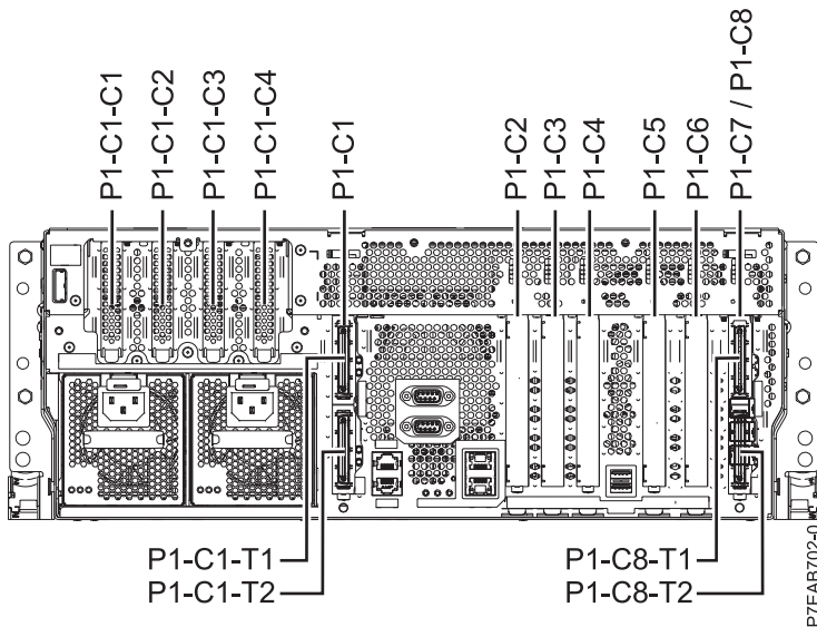
Figure 3. Vue arrière des systèmes 02E/4C et 05E/6C, montrant les emplacements PCI avec leurs codes d'emplacement
