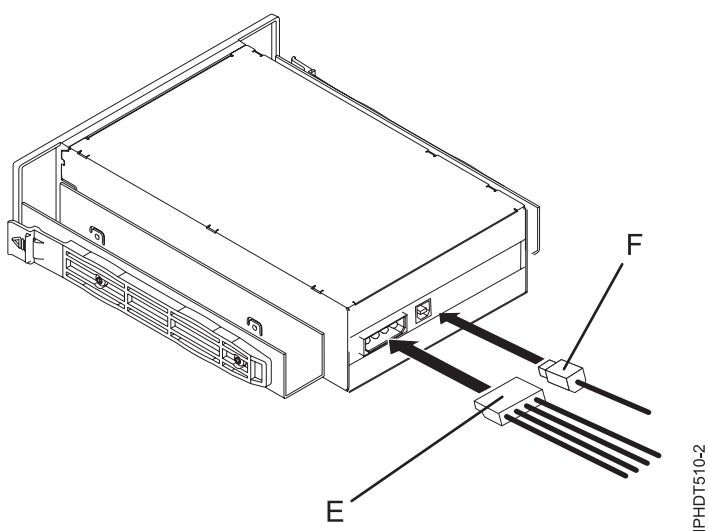
Figure 15. Unité interne, vue arrière et connecteurs
