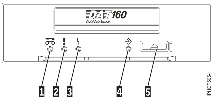
Figure 12. Vue avant de l'unité de bande
