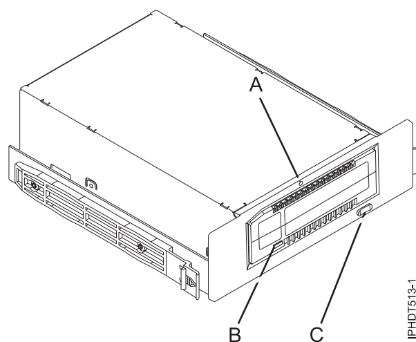
Figure 13. Unité interne, vue de face
