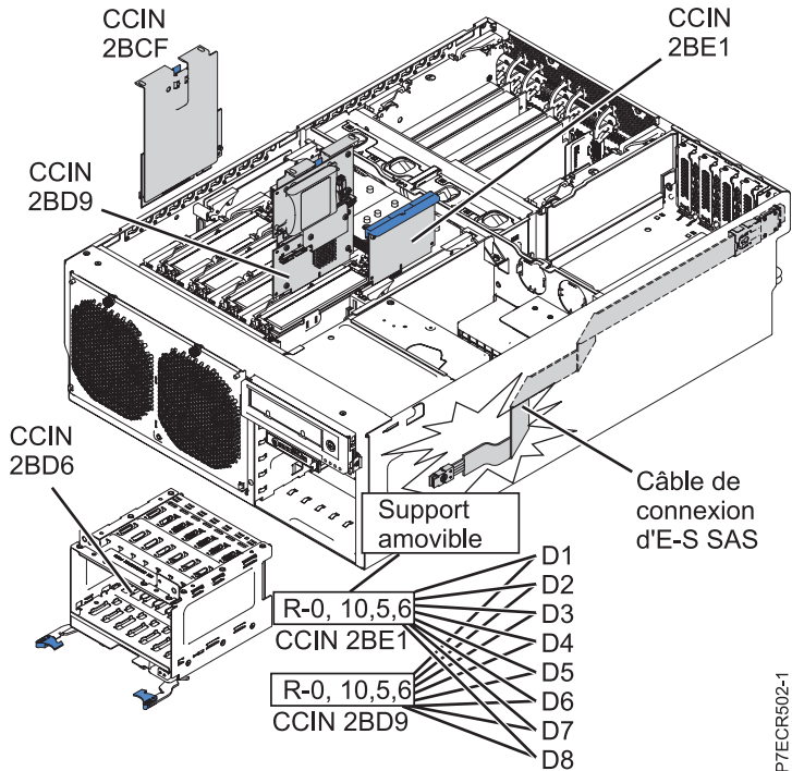
Figure 7. Baies de disques contrôlées par les deux adaptateurs SAS intégrés lors de l'utilisation d'un sous-système SAS RAID double avec unités externes
