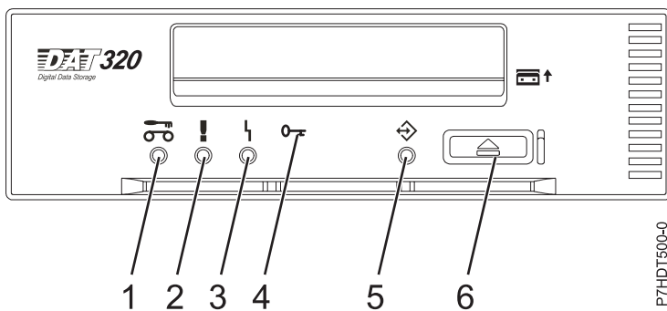
Figure 10. Vue avant de l'unité de bande
