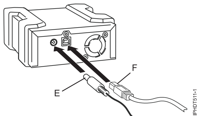
Figure 15. Unité externe, vue arrière et connecteurs
