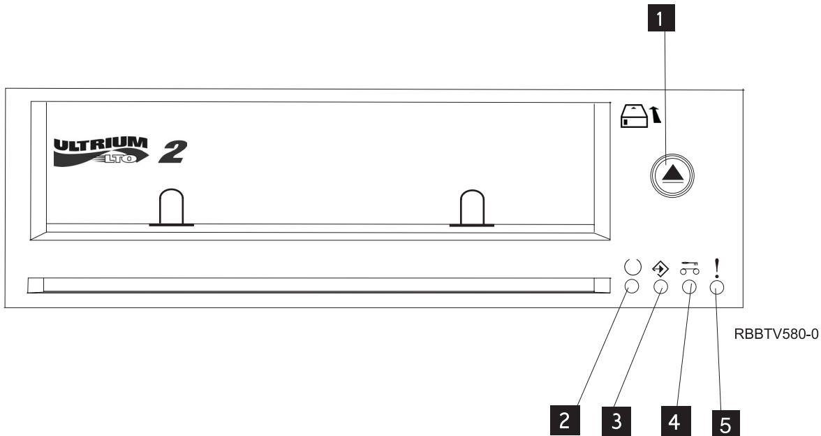
Figure 3. Vue avant de l'unité de bande
