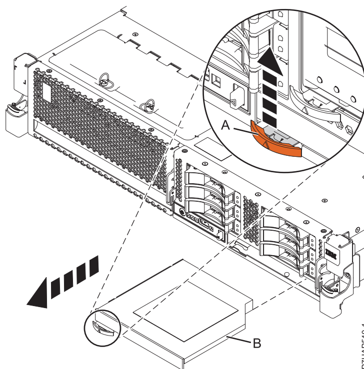
Figure 6. Retrait d'une unité de stockage extra-plate
