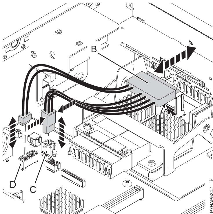
Figure 3. Connexions de câbles
