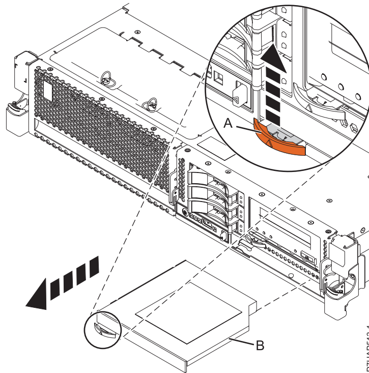
Figure 4. Retrait d'une unité de stockage extra-plate
