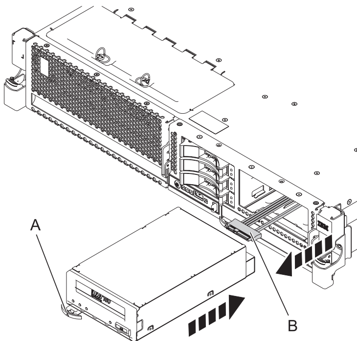
Figure 2. Installation d'une unité de stockage SAS
