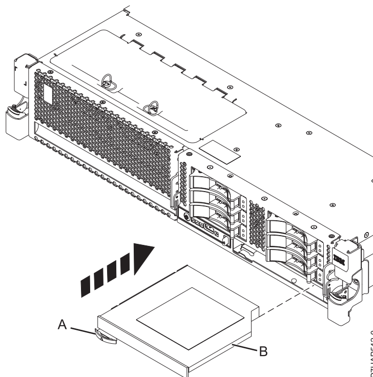
Figure 10. Installation d'une unité de stockage extra-plate
