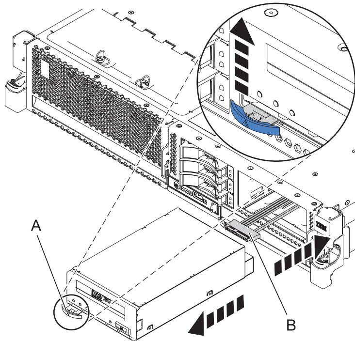
Figure 1. Retrait d'une unité de stockage SAS
