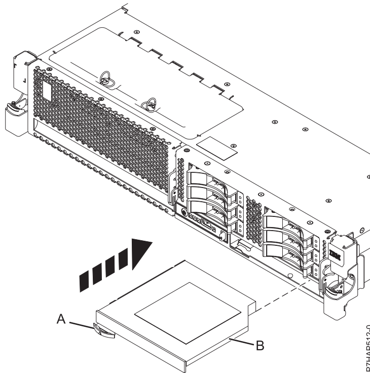
Figure 7. Installation d'une unité de stockage extra-plate
