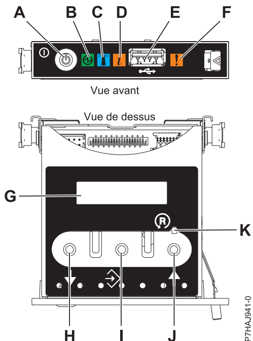
Figure 17. Panneau de commande
