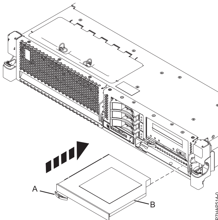
Figure 5. Installation d'une unité de stockage extra-plate
