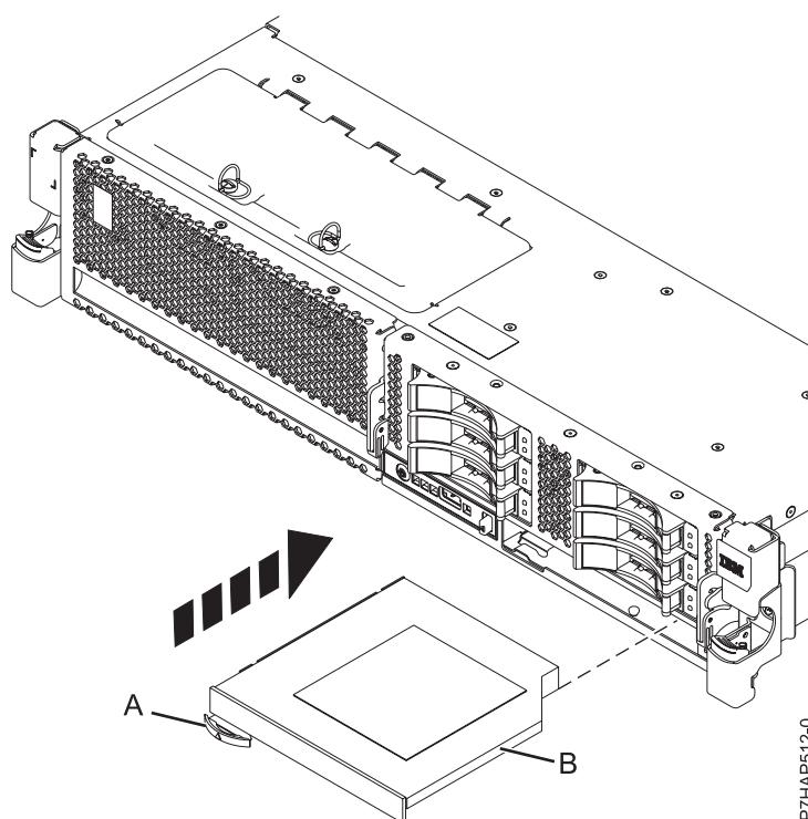
Figure 8. Installation d'une unité de stockage extra-plate
