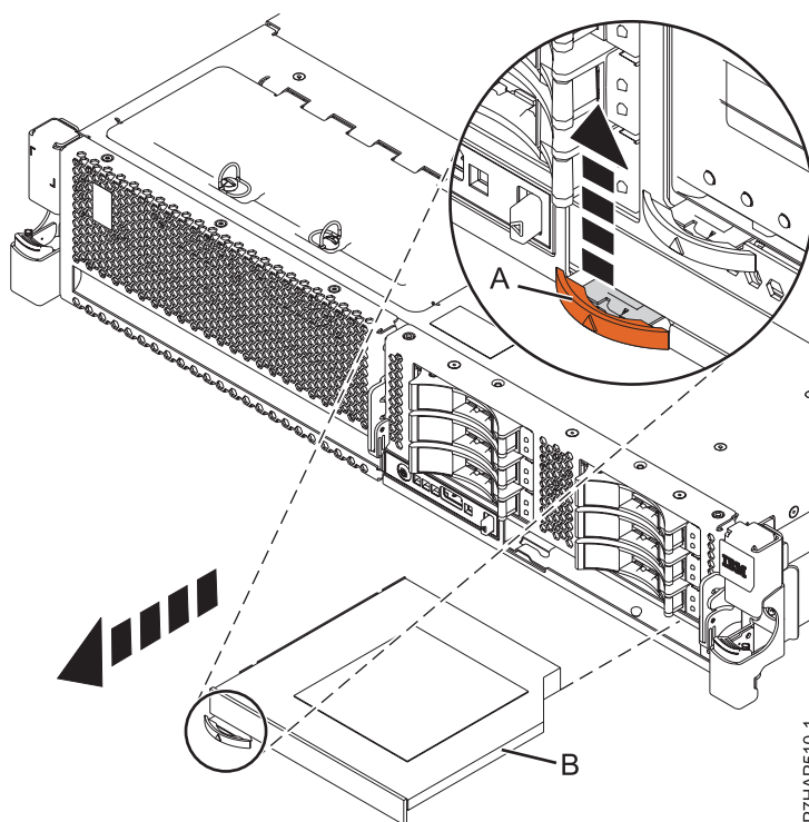
Figure 9. Retrait d'une unité de stockage extra-plate
