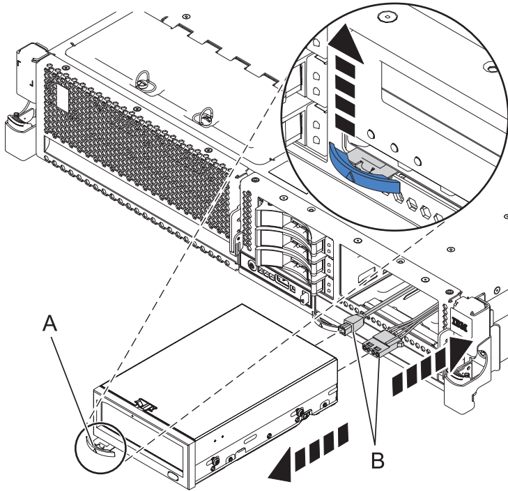
Figure 12. Retrait de l'unité de stockage
