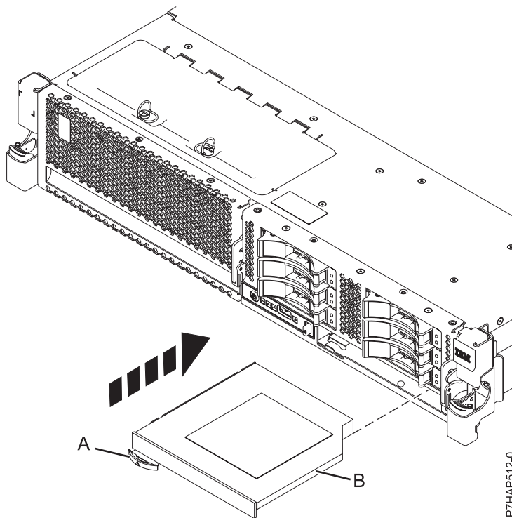
Figure 11. Installation d'une unité de stockage extra-plate
