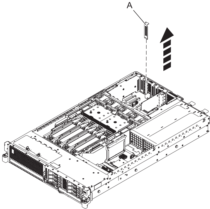
Figure 4. Retrait du panneau obturateur ou de la carte PCI d'une unité centrale montée en armoire
