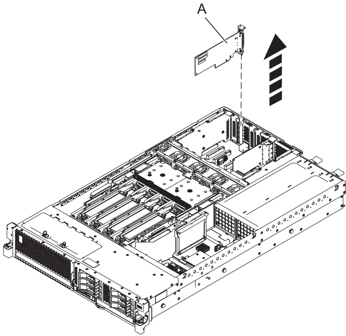
Figure 3. Retrait de la carte PCI d'une unité centrale montée en armoire
