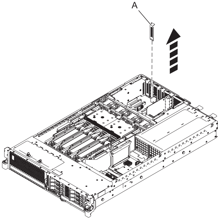
Figure 1. Retrait du panneau obturateur ou de la carte PCI d'une unité centrale montée en armoire
