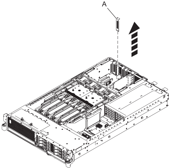
Figure 6. Retrait du panneau obturateur ou de la carte PCI d'une unité centrale montée en armoire
