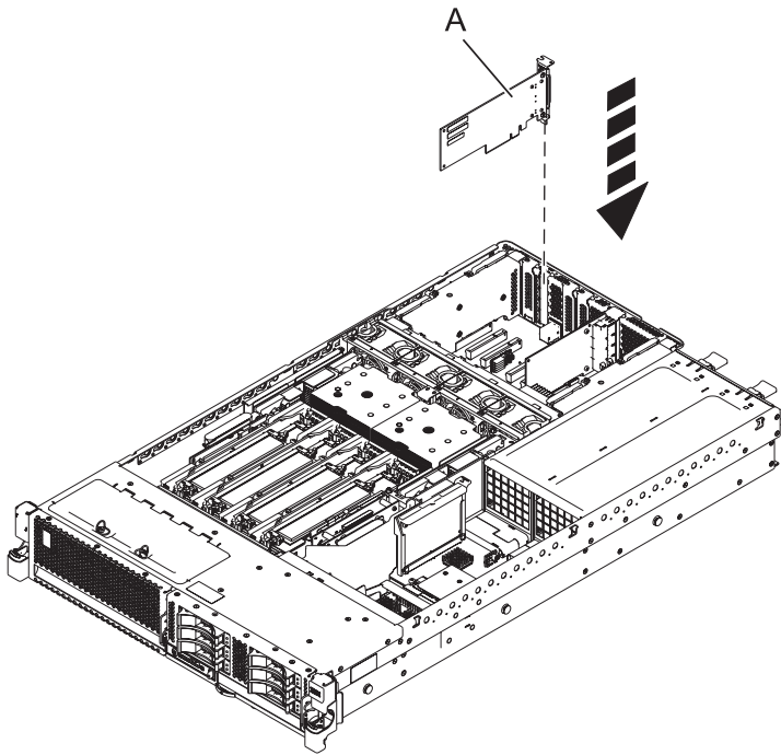
Figure 5. Remplacement de la carte PCI d'une unité centrale montée en armoire
